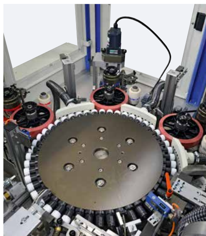
3 colores = 3 unidades de impresión rotativas por tampografía incorporados V-RTI 3000
