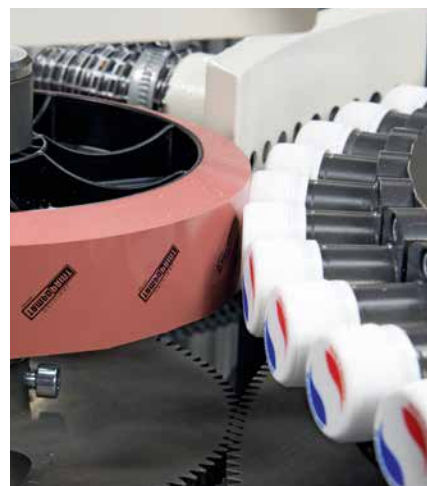
Las superficies irregulares no presentan problema, se puede imprimir sobre puntos de moldeo por inyección
